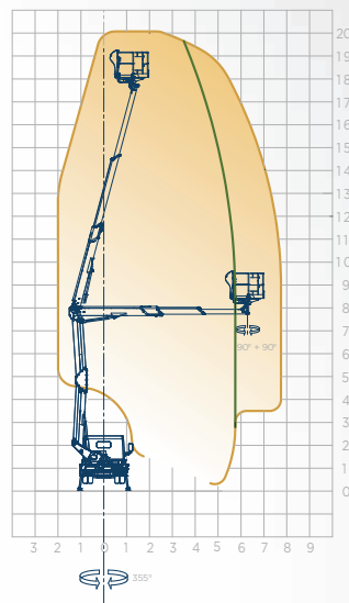
Stabilizzatori chiusi Closed outriggers
