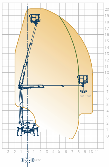
Stabilizzatori aperti Open outriggers
